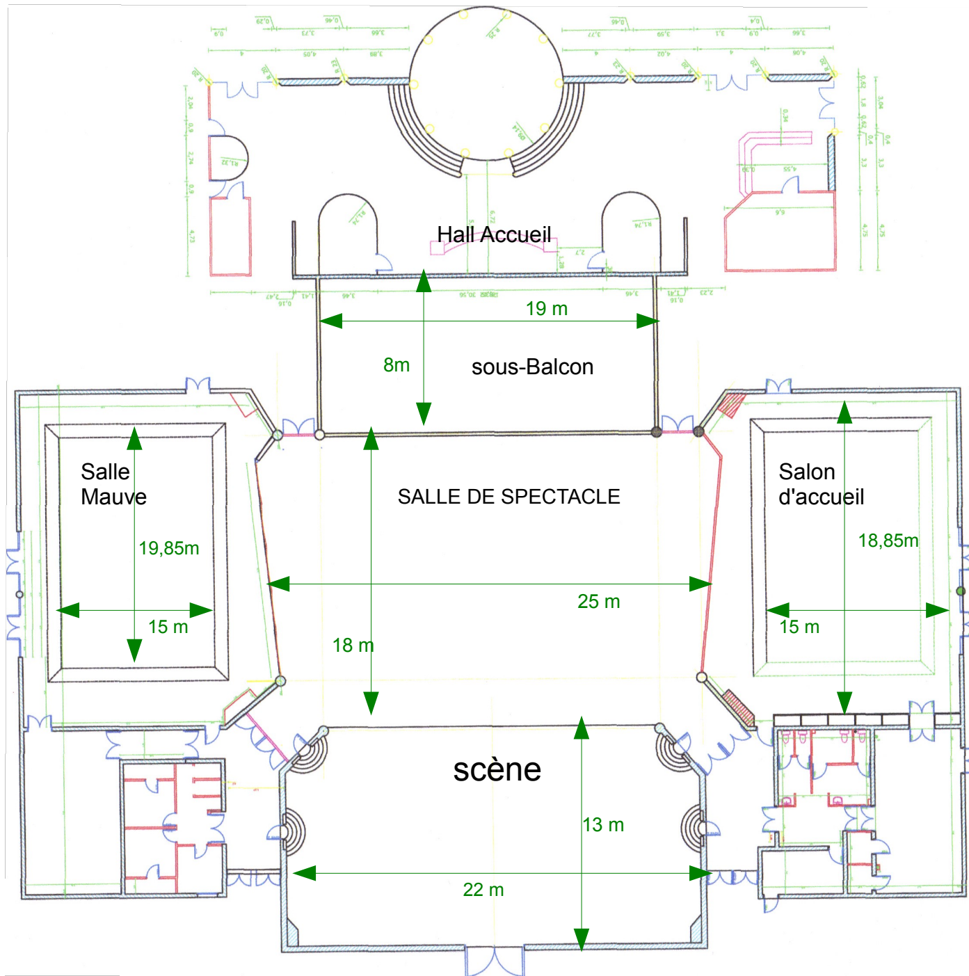
PLAN DE MASSE LA COUPOLE
